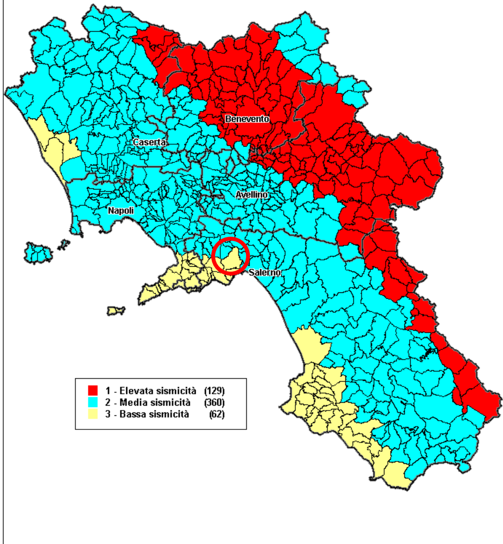
Classificazione sismica
