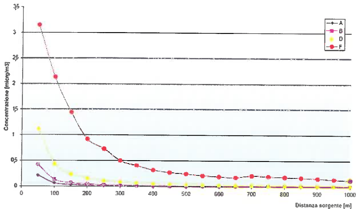
Figura 4.3.2.1. - Stima delle dispersioni di polveri in atmosfera in fase di costruzione al variare della classe di stabilità
