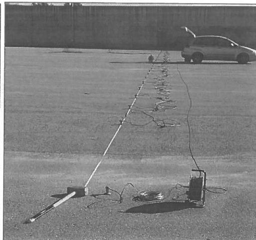
Stendimento indagine sismica Masw
