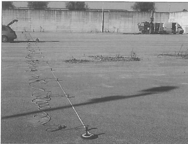
Stendimento indagine sismica Masw
