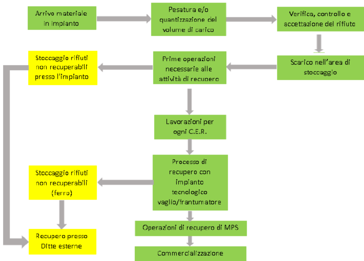
Figura 6: Diagramma di flusso del ciclo di produzione.
