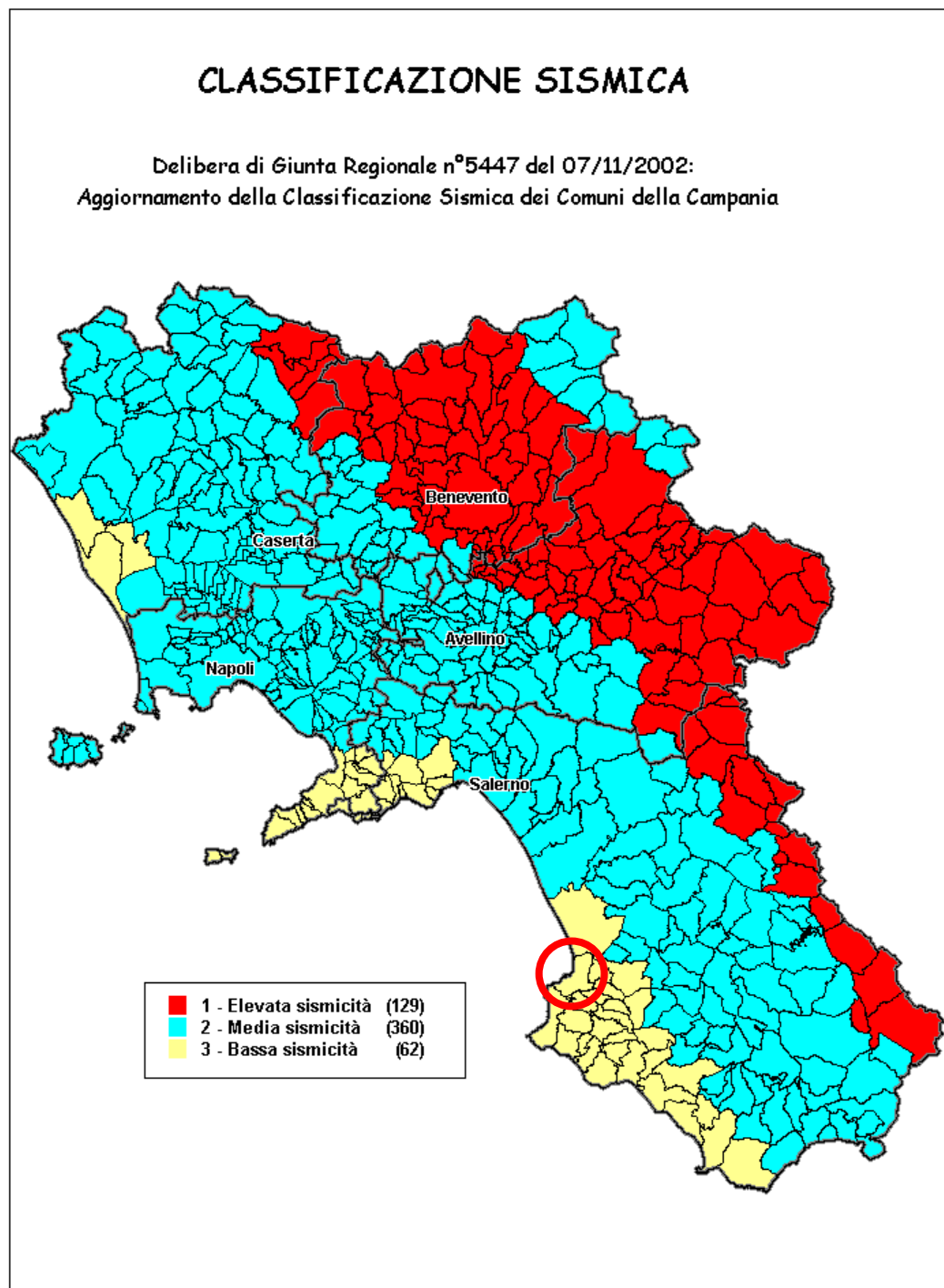
Classificazione sismica
